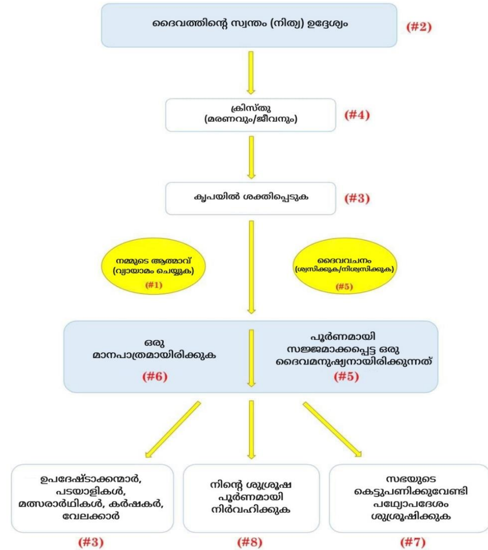
2024 ITERO-S ദൃതുകളുടെ ഒരു ഉദാഹരണ രേഖാചിത്രം
